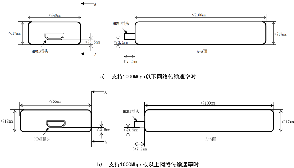
图1 直插式机顶盒尺寸和HDMI 插头位置
